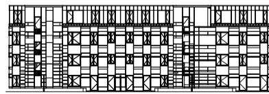
achtergevel
