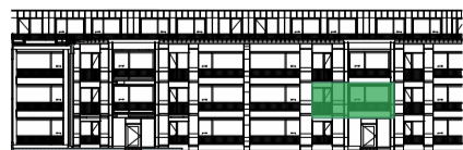
voorgevel
